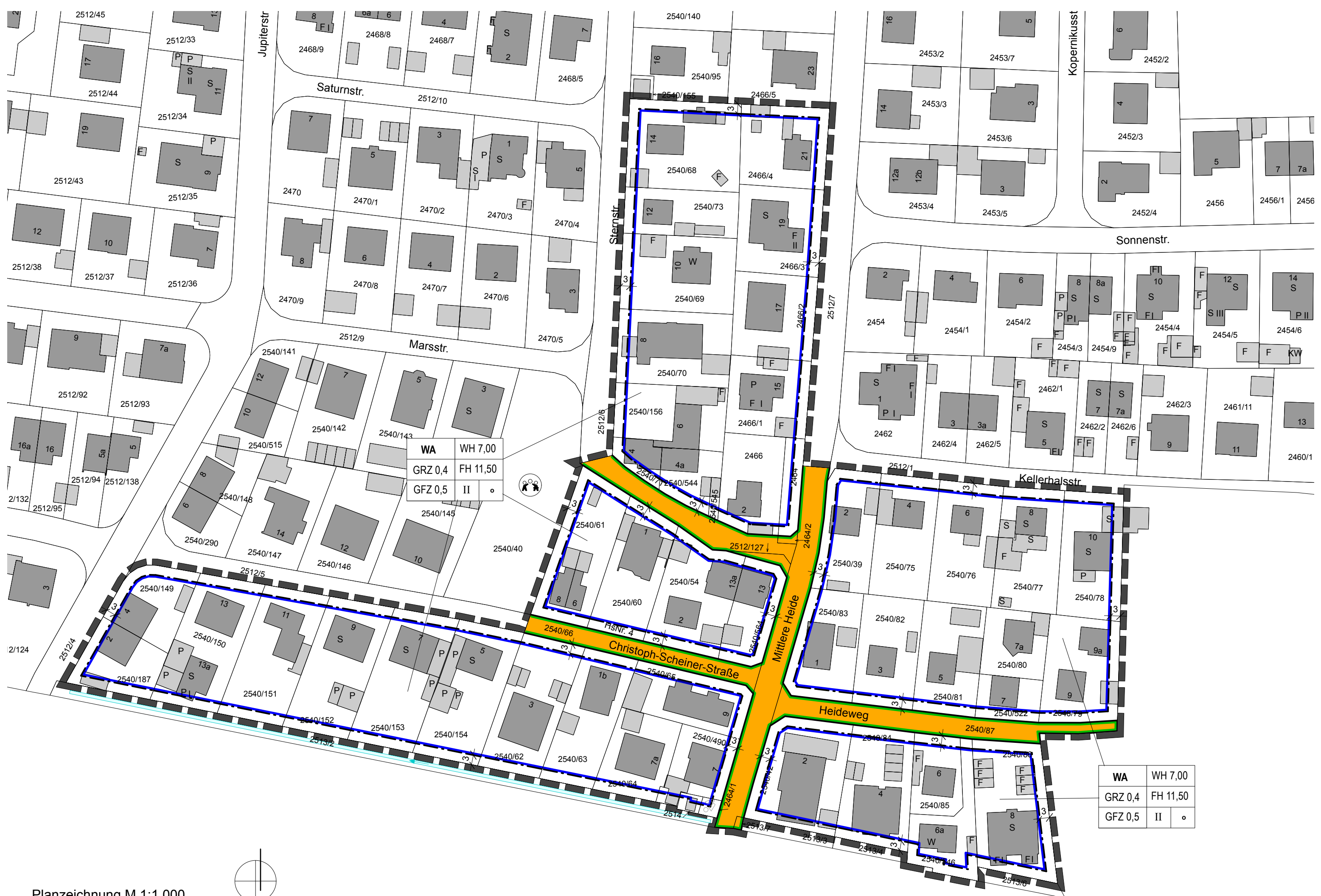
Planzeichnung M 1:1.000
